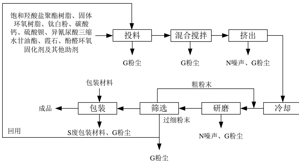
图 2.2-4 粉末涂料生产工艺流程
