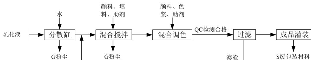
图 2.2-1 水性涂料生产工艺流程图
