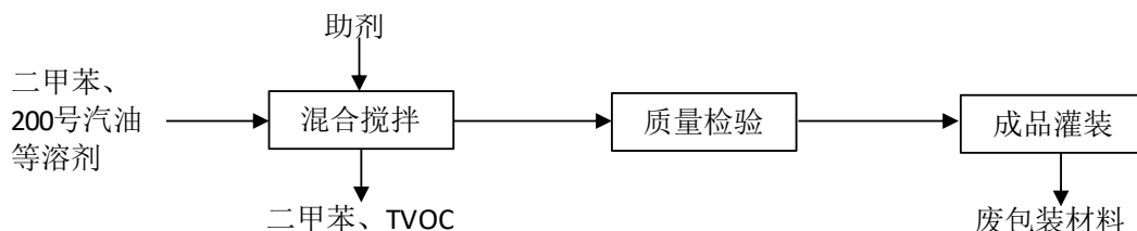
图 2.2-2 溶剂型涂料一般生产工艺流程图
