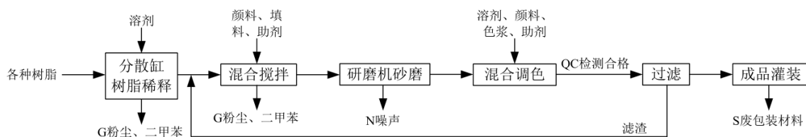
图 2.2-2 溶剂型涂料一般生产工艺流程图
